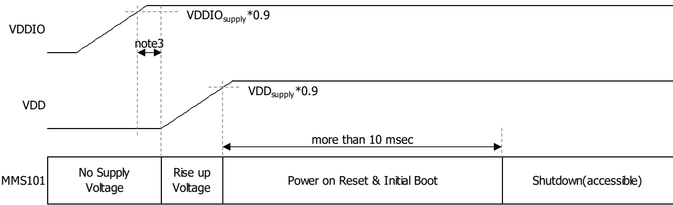
Fig. 5 電源投入シーケンス
