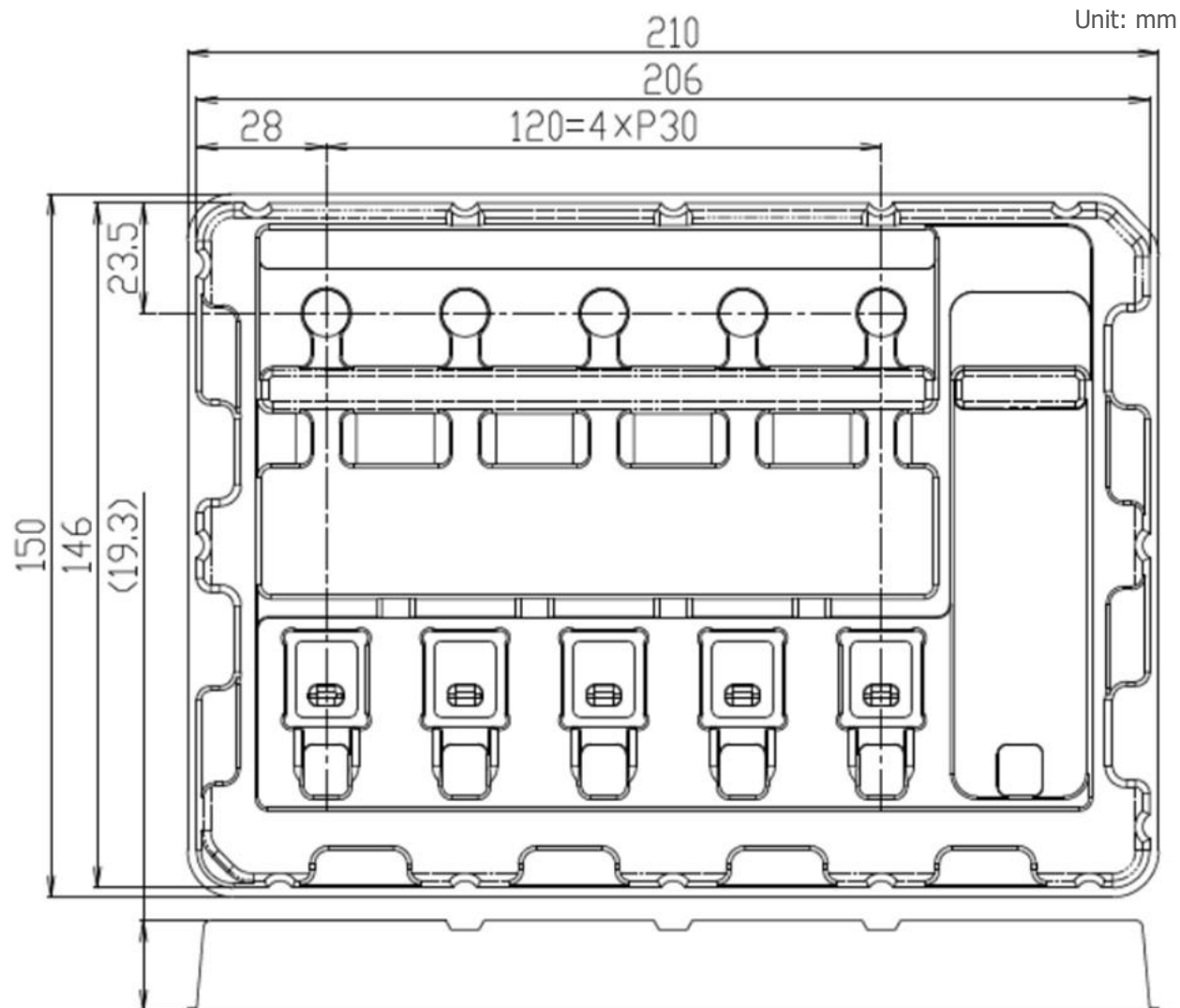
トレイ図面
