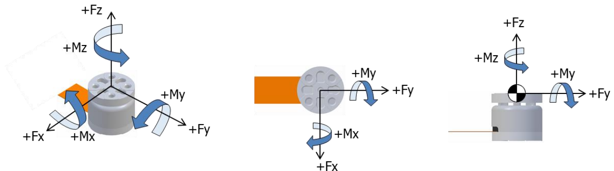
Fig. 28 座標系
