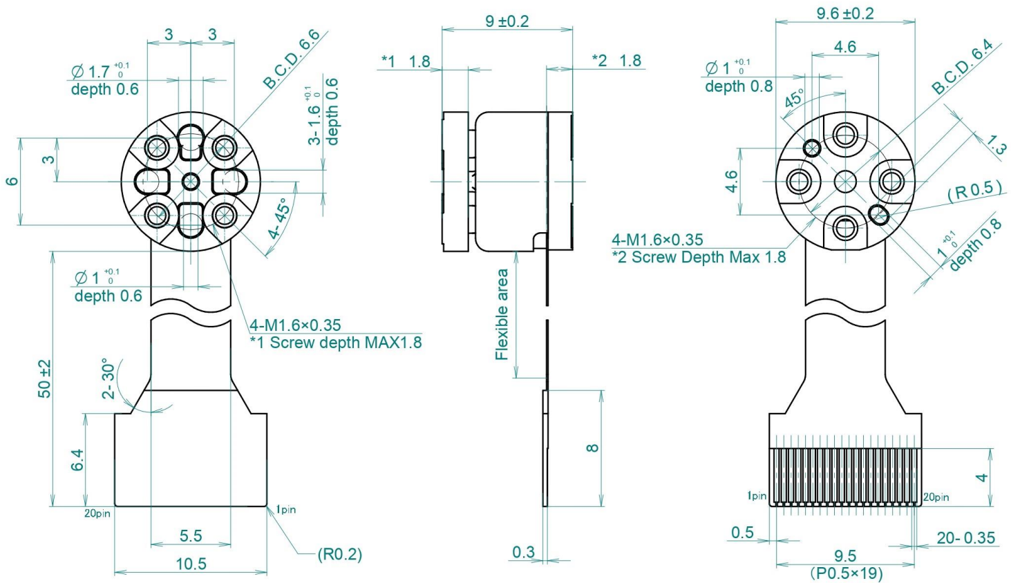
Fig. 27 外形図
