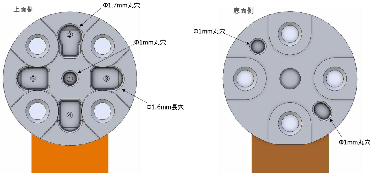
Fig. 35 位置決め穴
