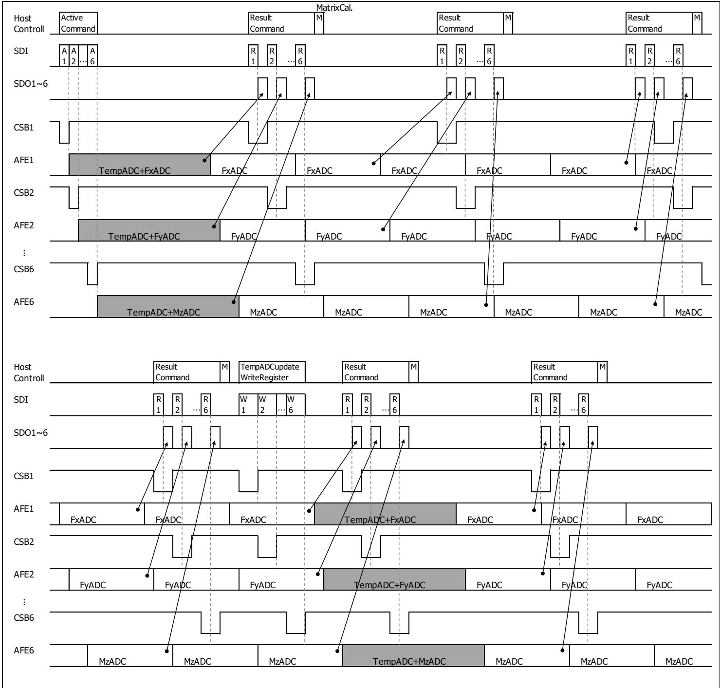
※各 AFE で内部クロックが異なる為、AD 変換の周期は各 AFE で異なります。 Fig. 18 SDO 端子共通 測定タイミング図
